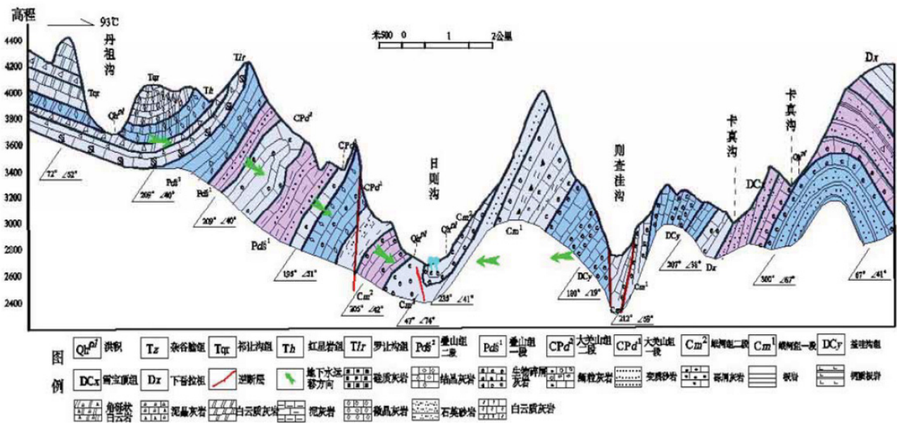
九寨沟景区水文地质剖面图(郑贵平, 2011)
