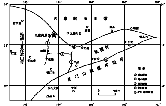
九寨溝景區所處大地構造位置圖(鄭貴平，2011)
