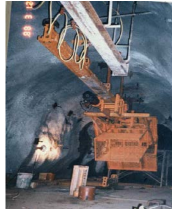
投影片7 壓力鋼管傾斜隧道導坑開挖之爬升機
